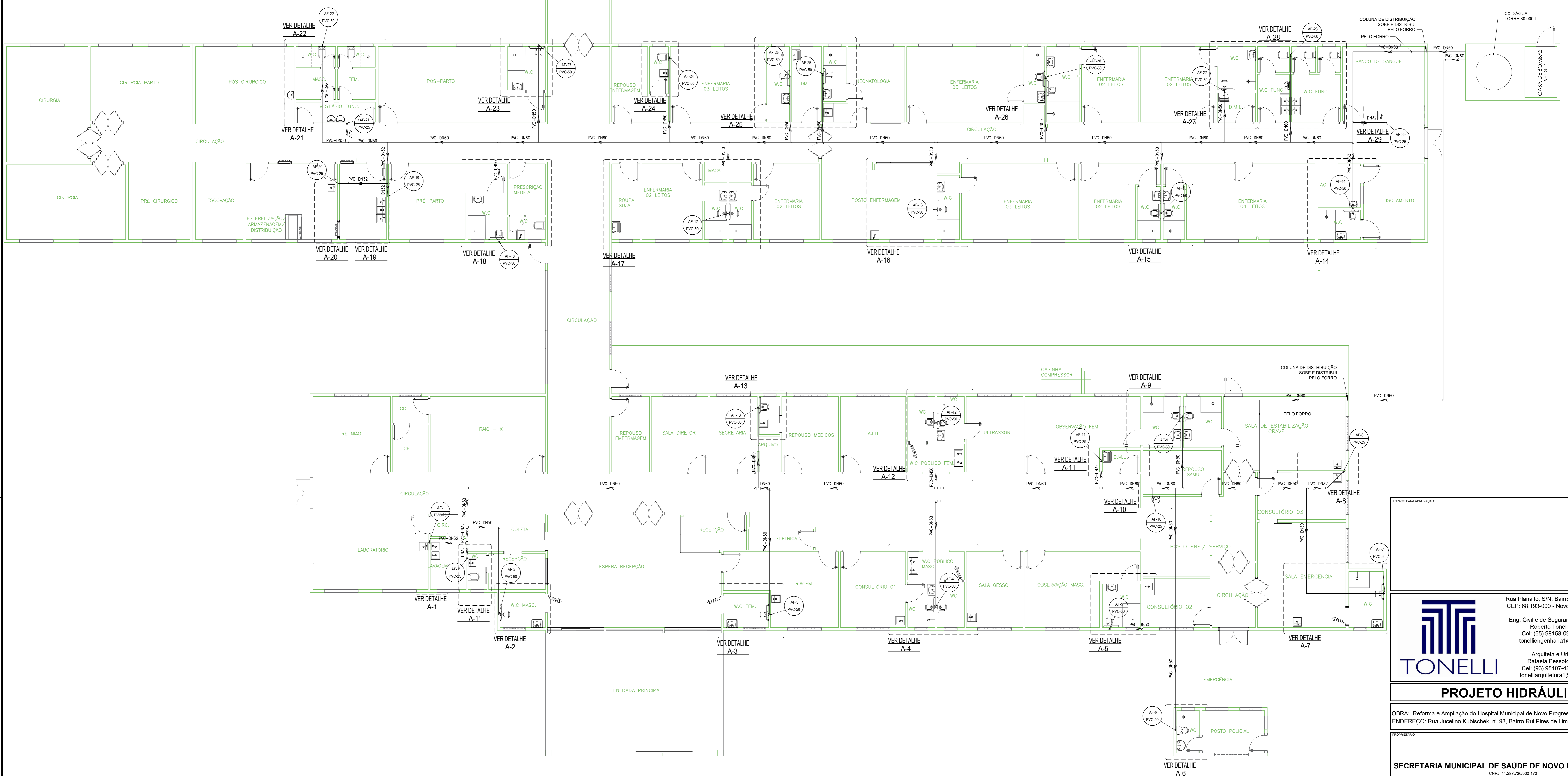
Planta Baixa - Implantação de distribuição de água escala 1:100 OBS: Reservatório de distribuição de água a pelo forro
