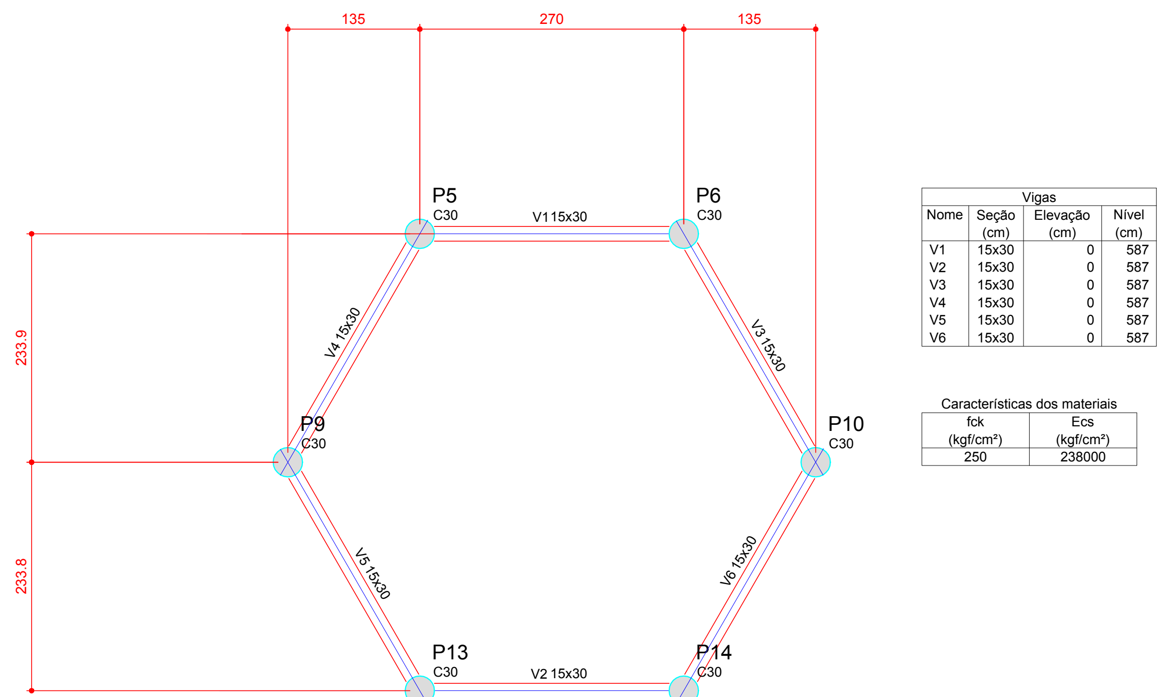
4 FORMA DO PAVIMENTO NÍVEL 587 ESCALA: 1/50
