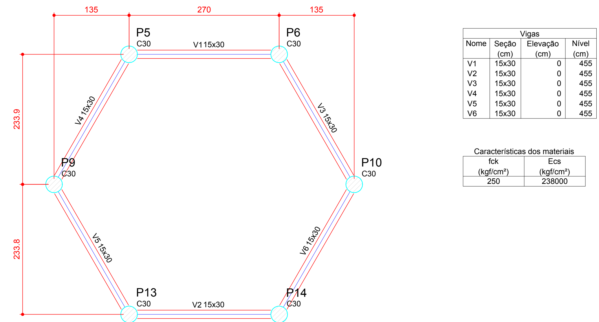
3 FORMA DO PAVIMENTO NÍVEL 455 ESCALA: 1/50
