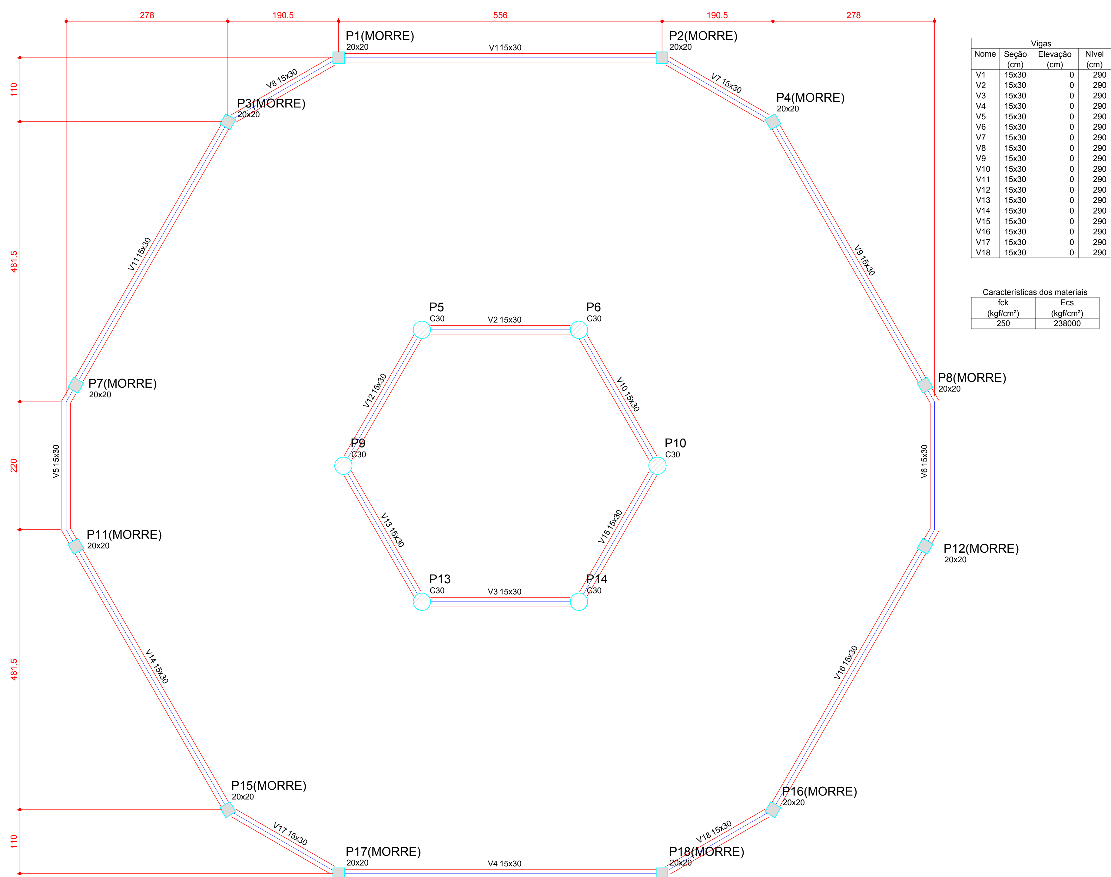
2 FORMA DO PAVIMENTO NÍVEL 290 ESCALA: 1/50
