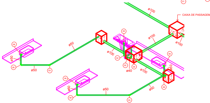
22 ISOMÉTRICO DETALHE 03 - SANITÁRIO
