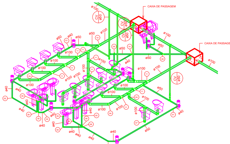
23 ISOMÉTRICO DETALHE 04 - SANITÁRIO
