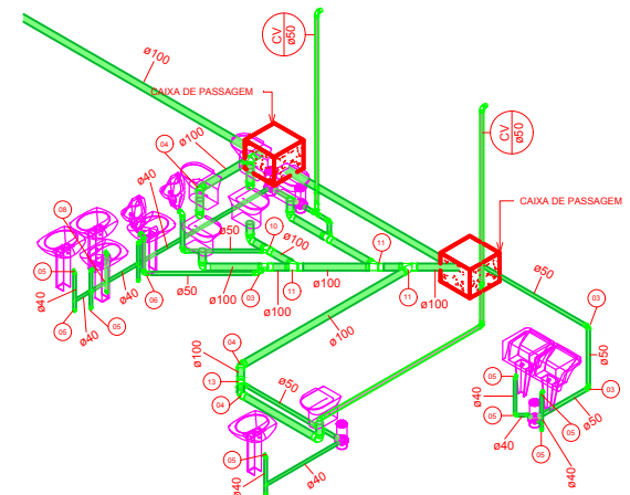
21 ISOMÉTRICO DETALHE 02 - SANITÁRIO
