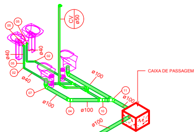
24 ISOMÉTRICO DETALHE 05 - SANITÁRIO
