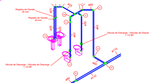
19 ISOMÉTRICO DETALHE 05 - HIDRÁULICO
