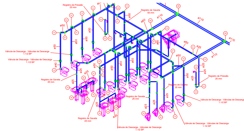
18 ISOMÉTRICO DETALHE 04 - HIDRÁULICO
