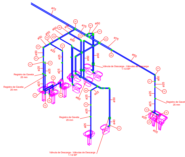
16 ISOMÉTRICO DETALHE 02 - HIDRÁULICO
