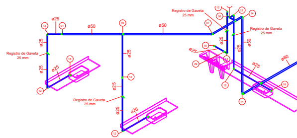
15 ISOMÉTRICO DETALHE 01 - HIDRÁULICO
