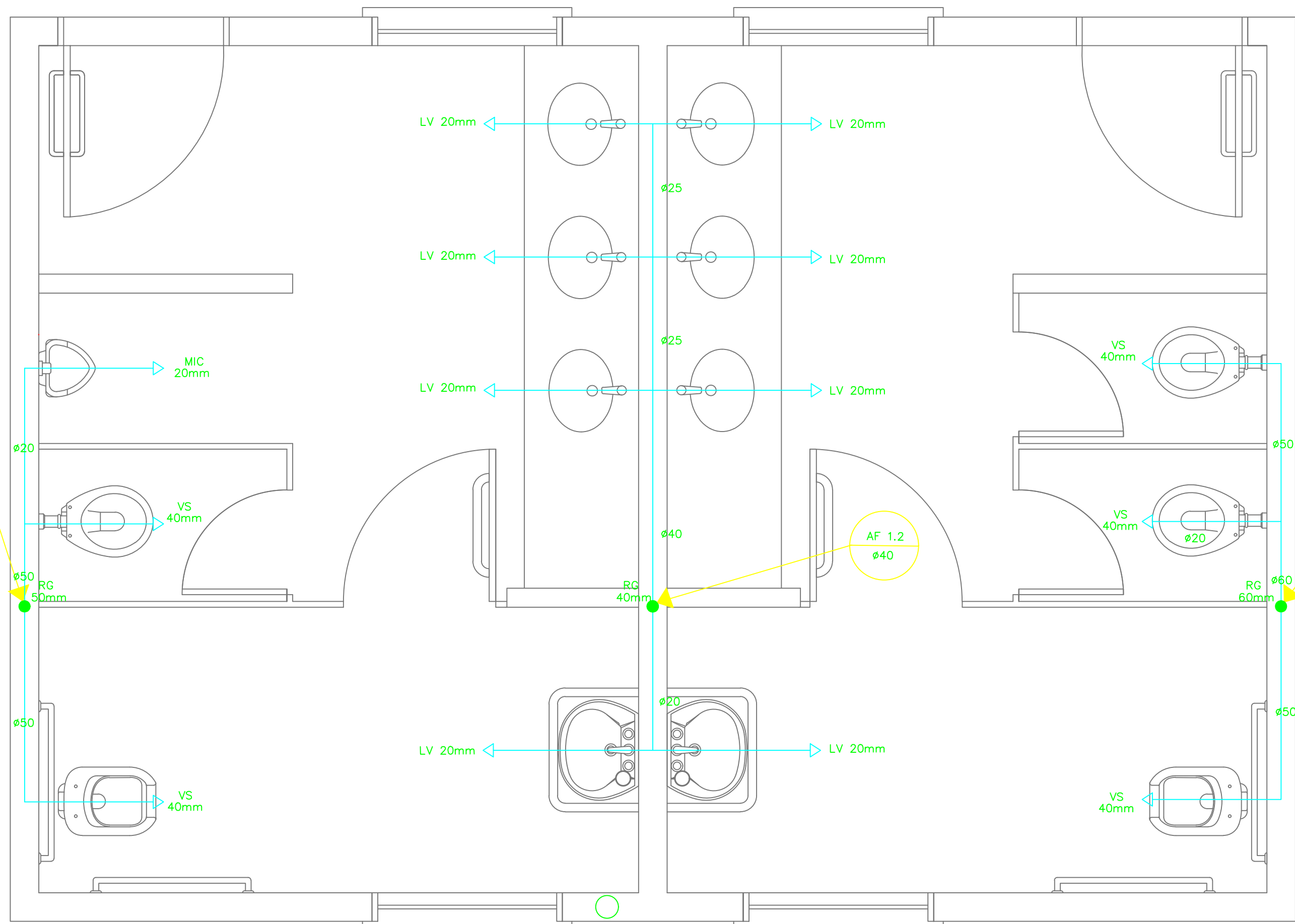
1 PLANTA BAIXA - SANITÁRIOS ALUNOS ESCALA 1/20
