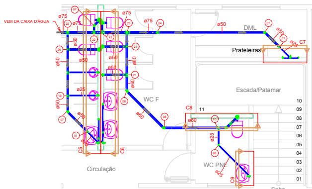
6 LAYOUT 02 - HIDRÁULICO 1 : 50
