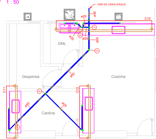
7 LAYOUT 03 - HIDRÁULICO 1 : 50
