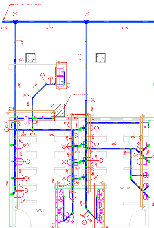
8 LAYOUT 04 - HIDRÁULICO 1 : 50
