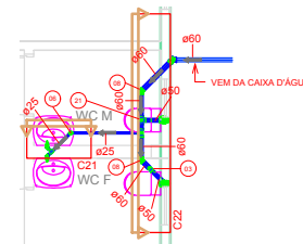
9 LAYOUT 05 - HIDRÁULICO 1 : 50
