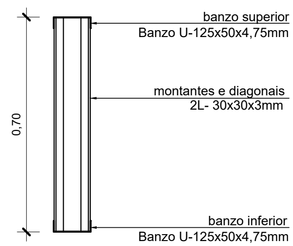
Seção da Tesoura Escala 1/25
