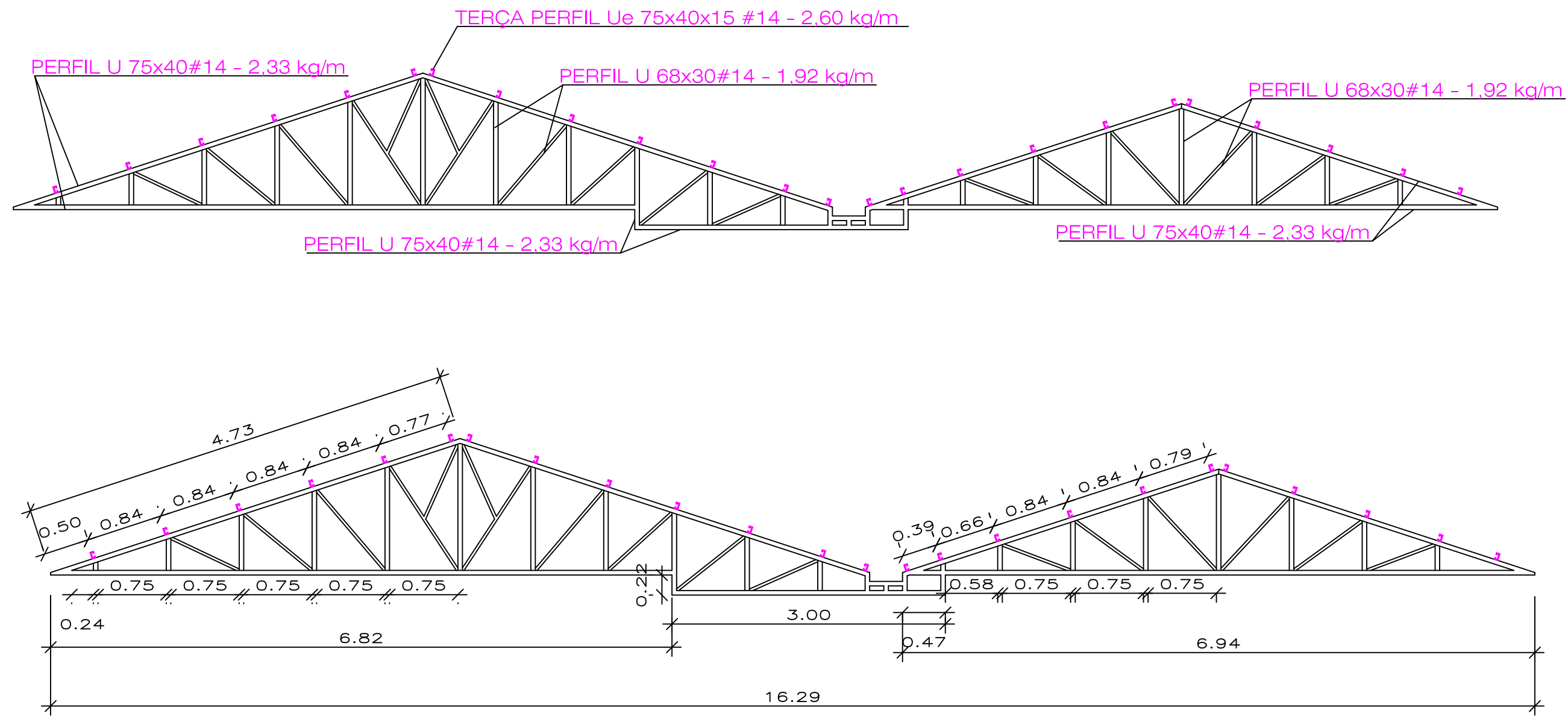
DET. DA TESOURA ESCALA: 1/50
