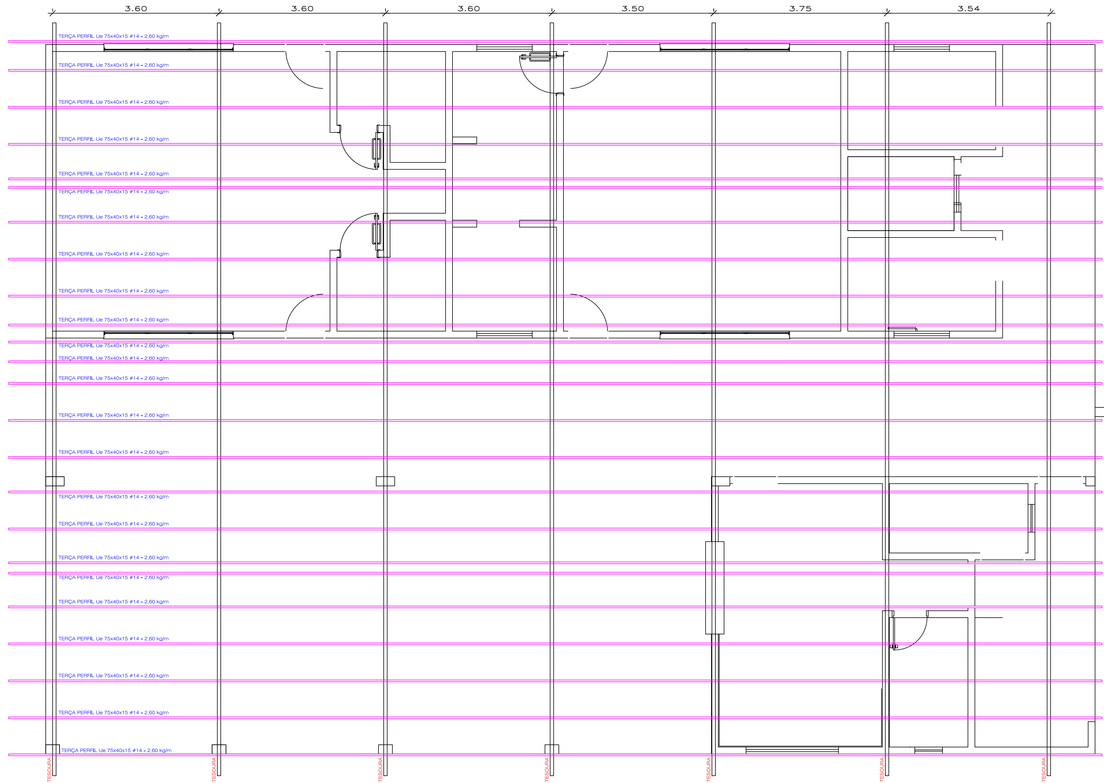
DISPOSIÇÃO DAS TESOURAS ESCALA: 1/50
