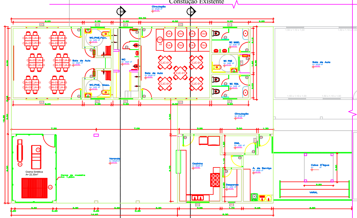
1 Planta Baixa Executiva Esc.: 1/50
