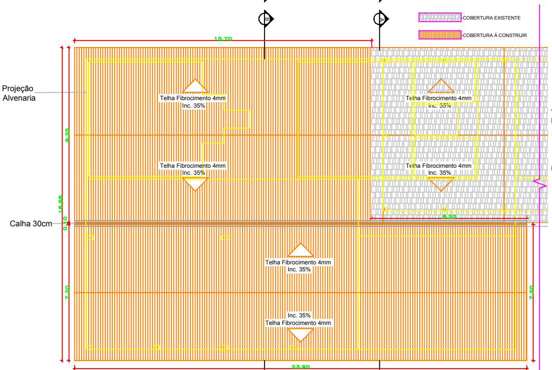
2 Planta de Cobertura Esc.: 1/50
