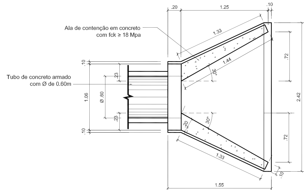
PLANTA BAIXA Boca de Bueiro simples de concreto Ø 0.60m
