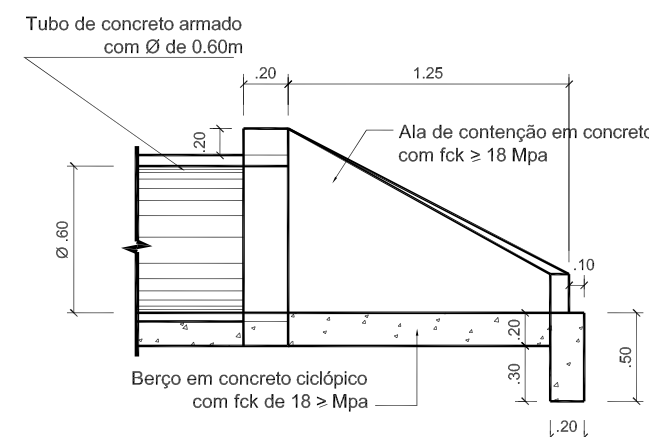
VISTA LATERAL Boca de Bueiro simples de concreto Ø 0.60m
