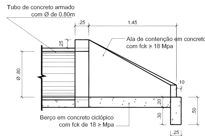
VISTA LATERAL Boca de Bueiro simples de concreto Ø 0.80m
