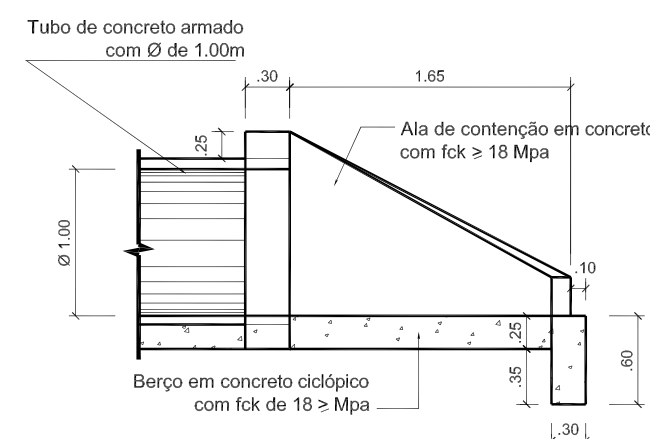
VISTA LATERAL Boca de Bueiro simples de concreto Ø 1.00m
