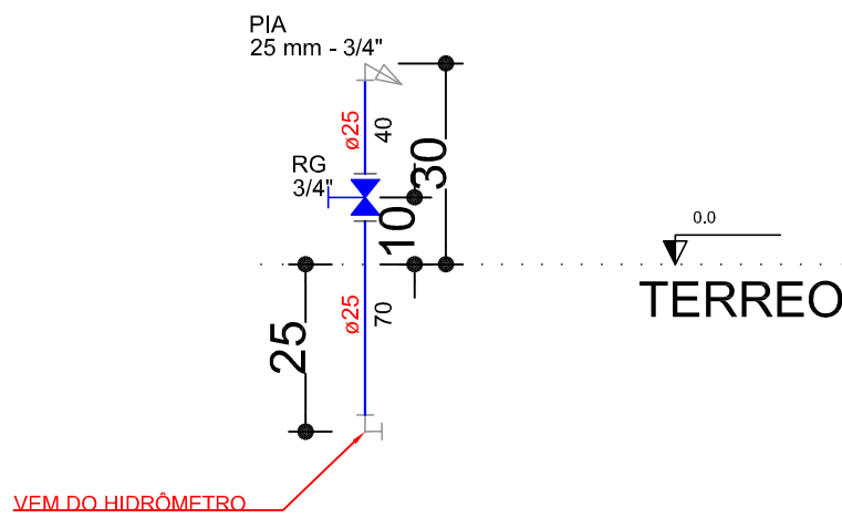
Corte C1 escala 1:25
