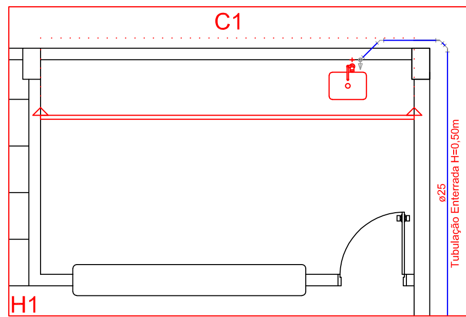
Planta Baixa escala 1:50
