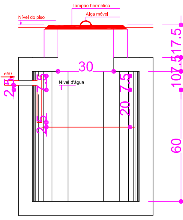
TANQUE SÉPTICO CORTE - ESC. 1:25
