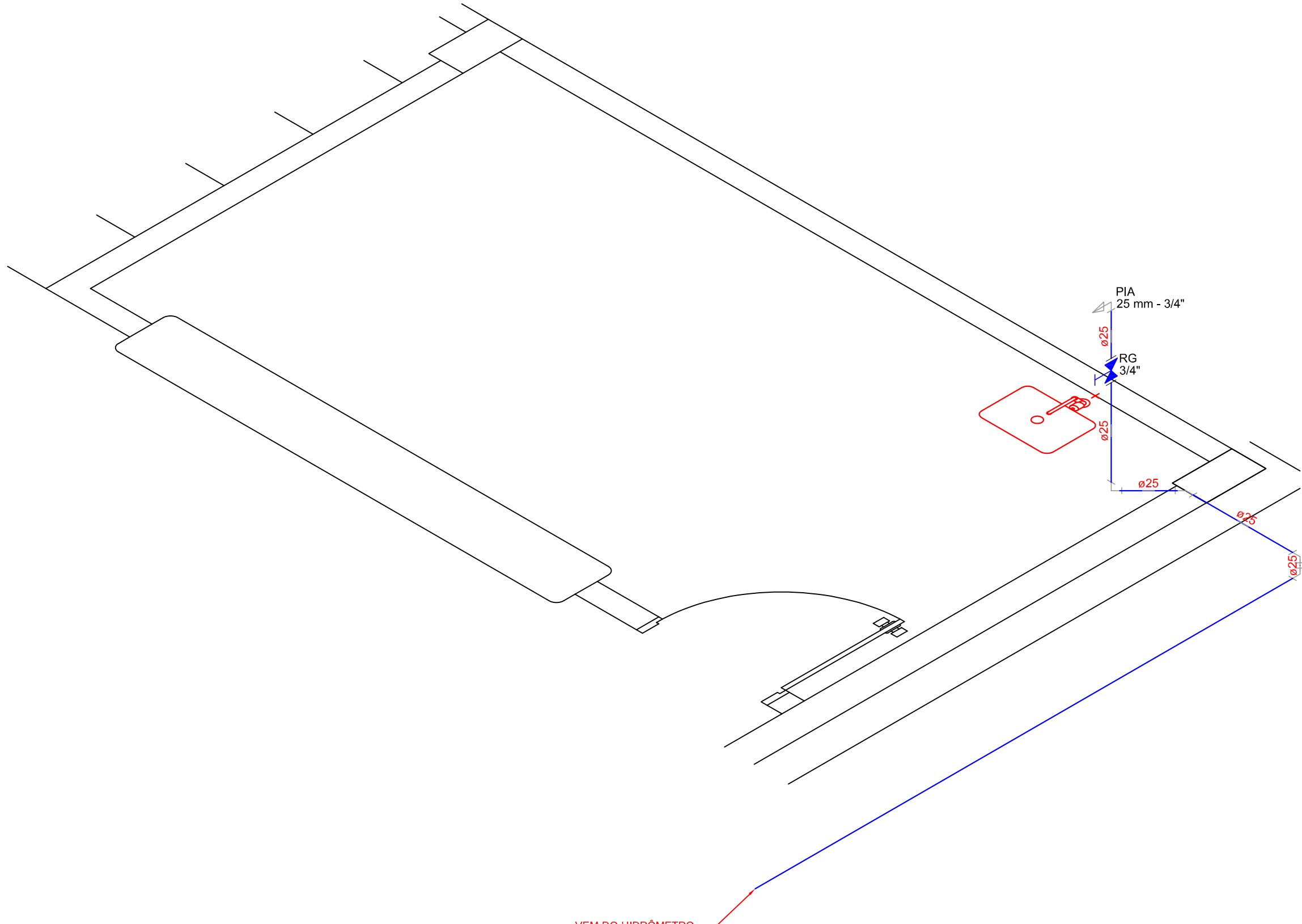
Detalhe H1 escala 1:25
